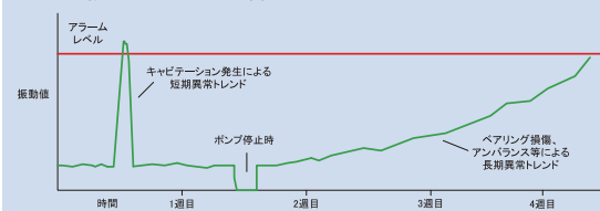
ポンプの振動トレンドデータ例
