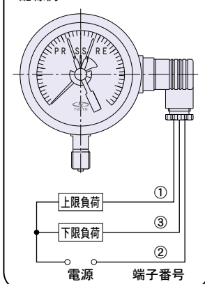
配線例
