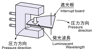
光電スイッチ構造図 Photo Switch Construction drawing
