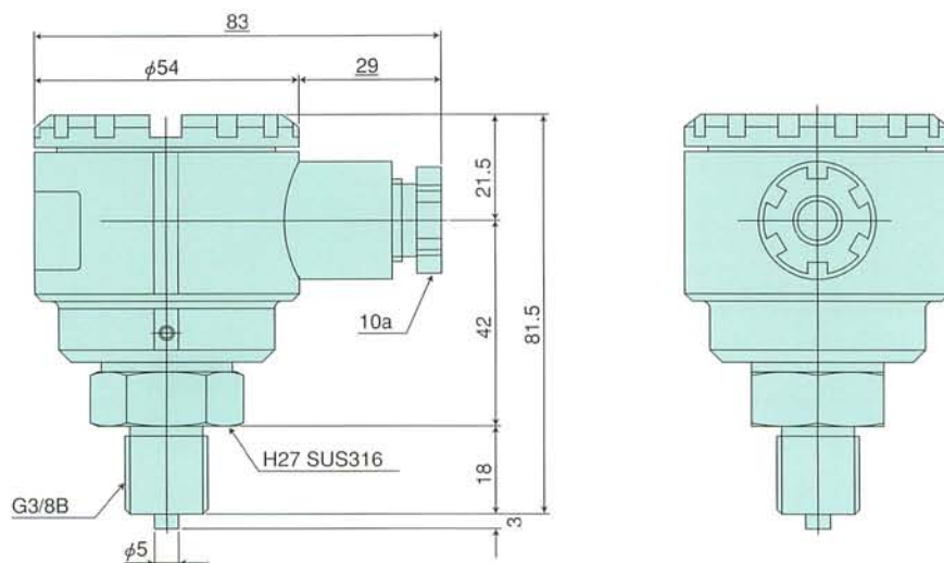
4～20mA式
