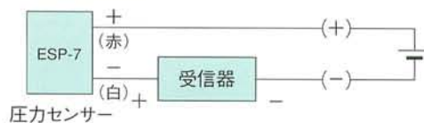
4～20mA式
